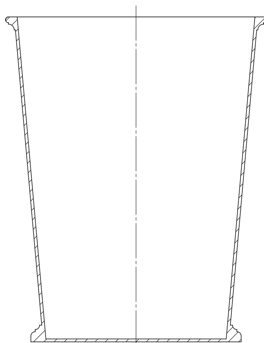
SECTION A-A
